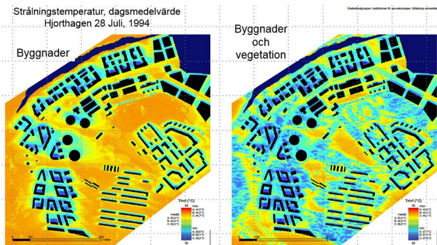
Modellering av strålningstemperatur, med och utan vegetation, Hjorthagen i juli 1994.
